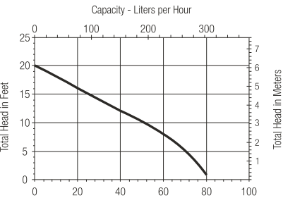
CP-MPG-115 / CP-MPG-115-T / CP-MPG-115-LP
